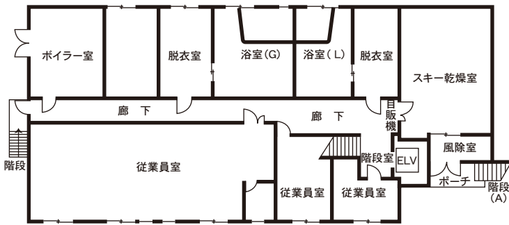
B1階 平面図
