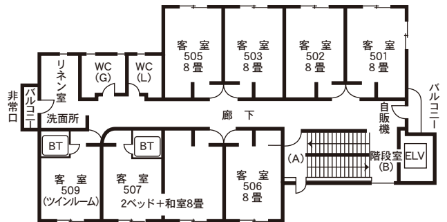
5階 平面図
