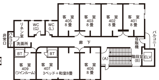
4階 平面図
