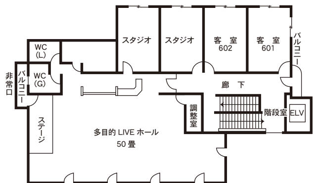
6階 平面図
